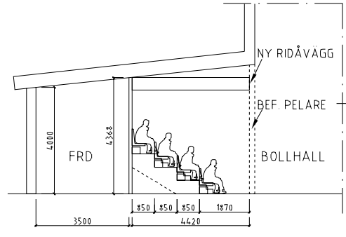
PRINCIPSEKTION LÄKTARE 1:100 (A1)
